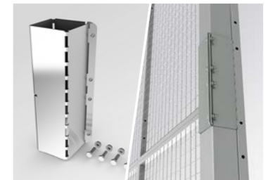
9 KOPPELSTUKKEN 80x80
