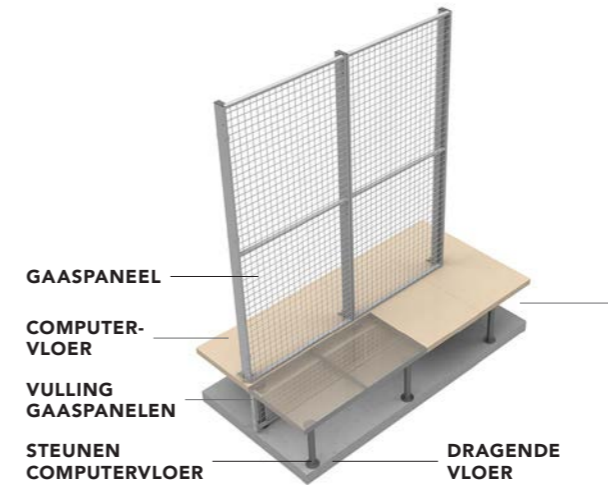
Een voorbeeld van een gaasvulling tussen de vaste vloer en de computervloer.
